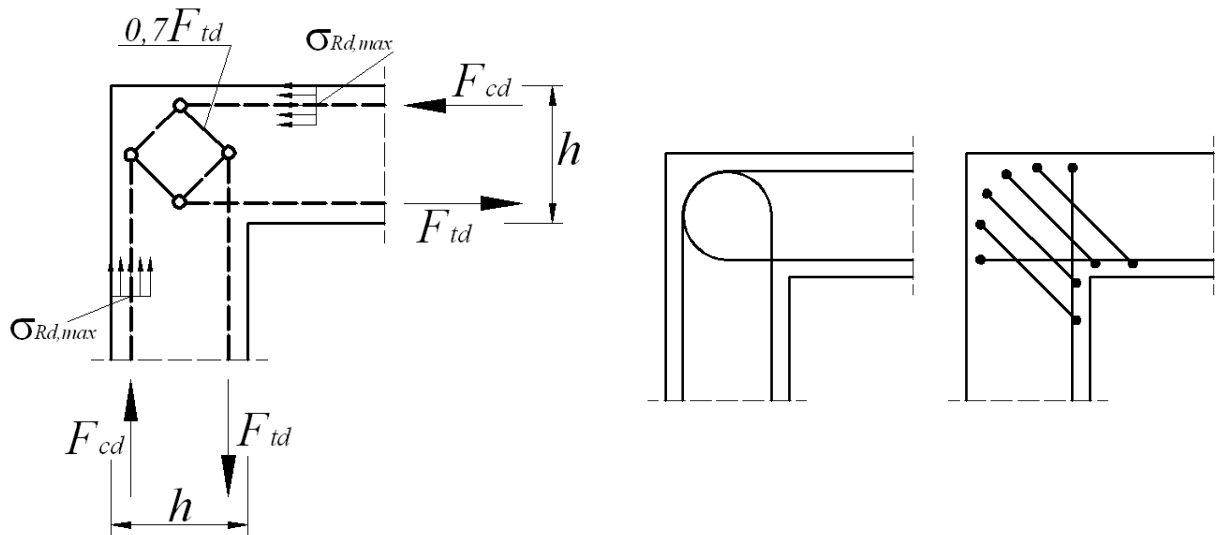
а) Модель «распорка и тяж»
