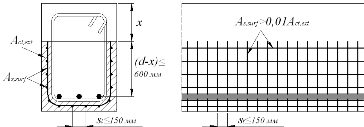
Рисунок Б.1 — Примеры поверхностной арматуры
