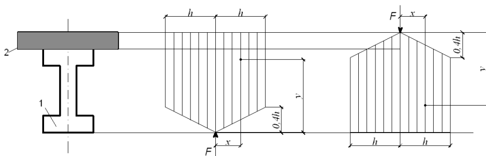
1 – сборный элемент; 2 – монолитный бетон
