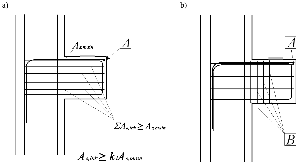
Рисунок Б.6 — Конструирование арматуры консоли: а — арматура при a_c \leq 0,5h_c б — арматура при a_c > 0,5h_c
