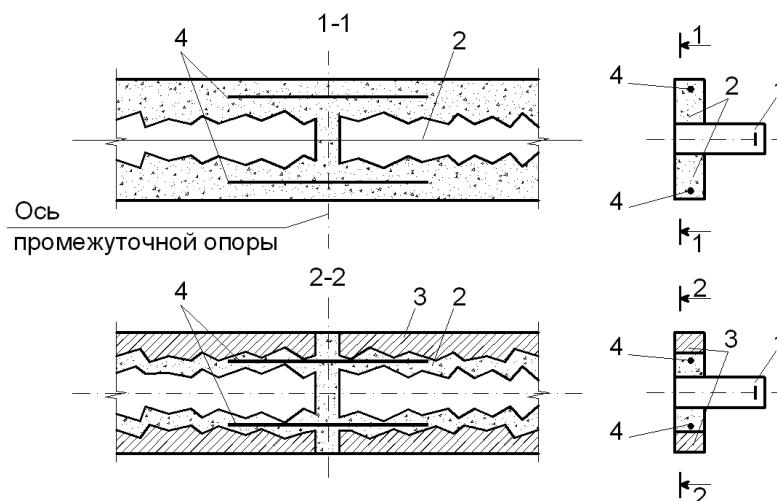
Рисунок 9.28 – Направление зубьев в сборных элементах статически неопределимых конструкций при вертикальных (наклонных) контактах
