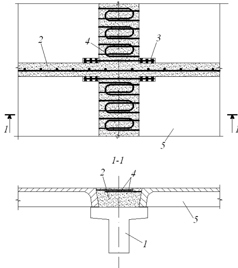
Рисунок 9.31 – Сопряжение плит
