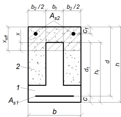
1 – сборный элемент; 2 – монолитный бетон
