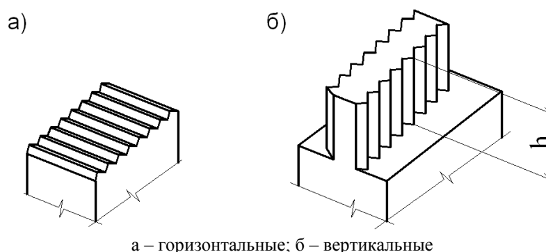
Рисунок 9.26 – Поперечные бетонные шпонки
