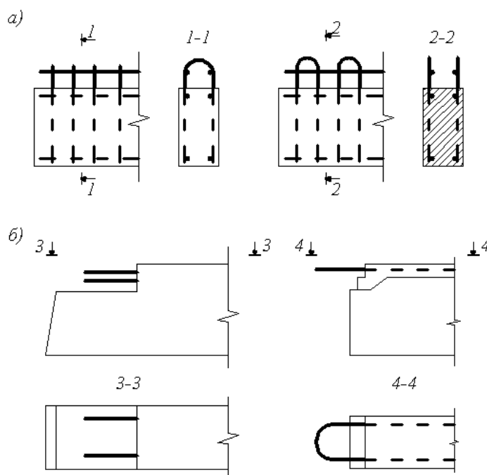
Рисунок 9.25 – Выпуски арматуры из сборных элементов
