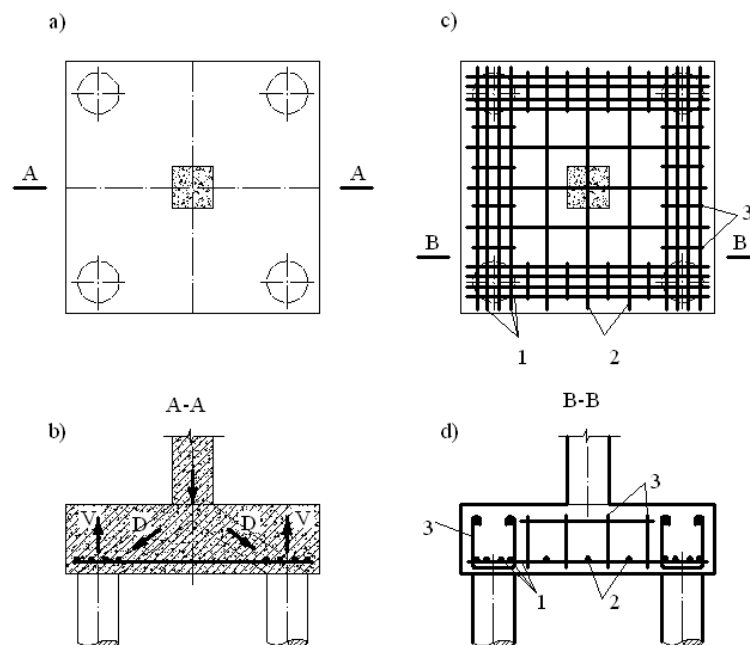
а – план; б – схема внутренних усилий; в – схема армирования; 1 - арматурные контурные пояса для восприятия распора; 2 – арматура центральной зоны ростверка; 3 – хомуты контурных поясов
