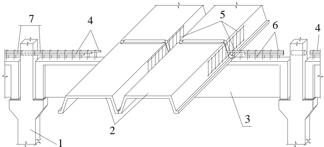
Рисунок 9.31 – Сопряжение плит
