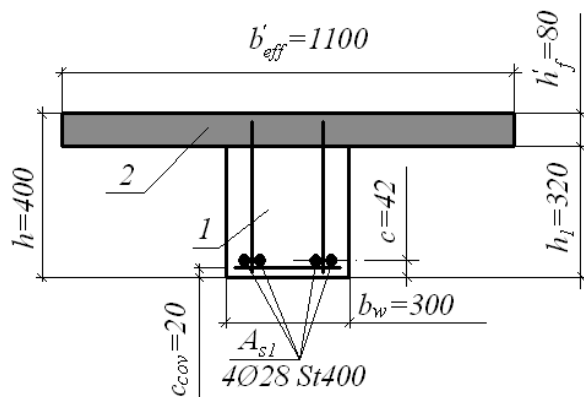
1 – сборный элемент; 2 – монолитный бетон
