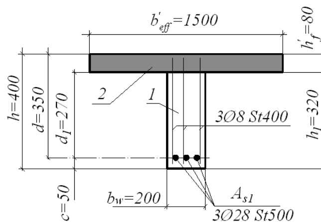
Рисунок Г.9. К расчету прочности наклонного сечения составной балки по сжатой полосе между трещинами.
