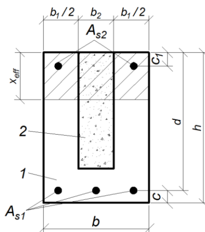
Рисунок 9.4 – Сечение элемента
