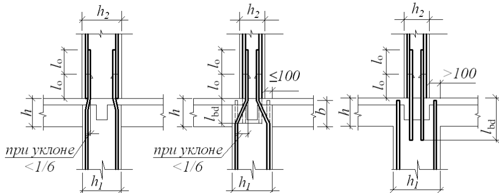
а – при одинаковом сечении колонн верхнего и нижнего этажей; б, в – при различии в сечениях колонн верхнего и нижнего этажей незначительном и резком соответственно
