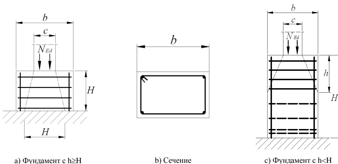
Рисунок 7.36 – Арматура, воспринимающая раскалывающие усилия, для фундамента на скальной породе
