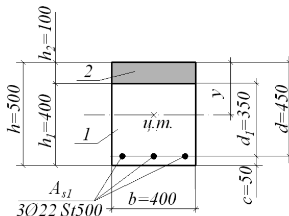
1- сборный элемент; 2 – монолитный бетон
