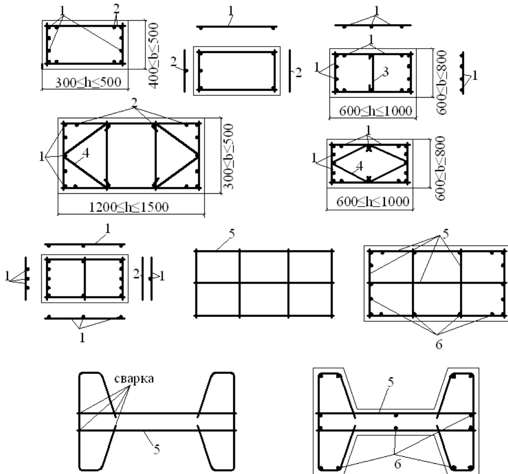
1- сетка; 2 – сетка или соединительный стержень; 3 – соединительный стержень (шпилька); 4 – хомут; 5 – поперечная арматура в виде сварной сетки; 6 – отдельные стержни продольной арматуры.
