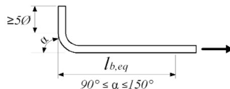
б) Эквивалентная длина анкеровки для стандартных 3 гибов
