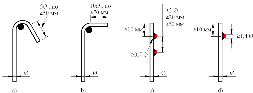
Рисунок 7.5 – Анкеровка хомутов
