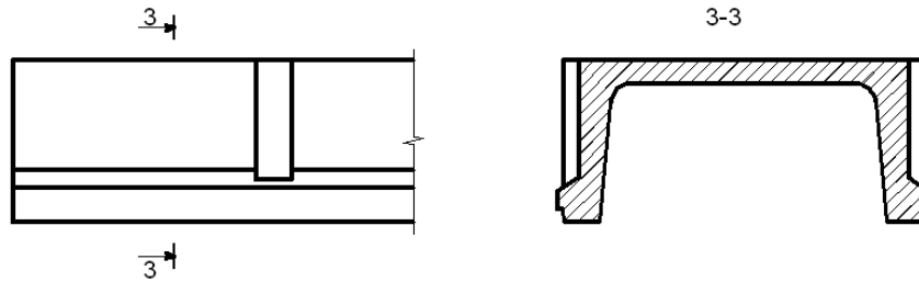
Рисунок 9.35 – Конструкции опорных участков сборных элементов
