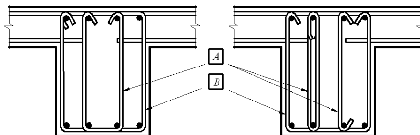
Рисунок 7.20 – Примеры поперечной арматуры
