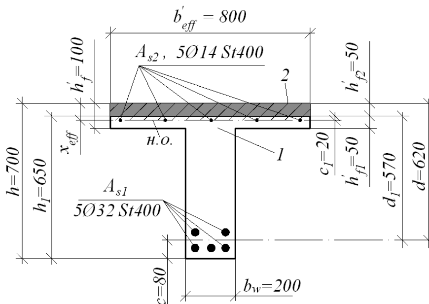
1 - сборный элемент таврового профиля с двойным армированием; 2 - набетонка
