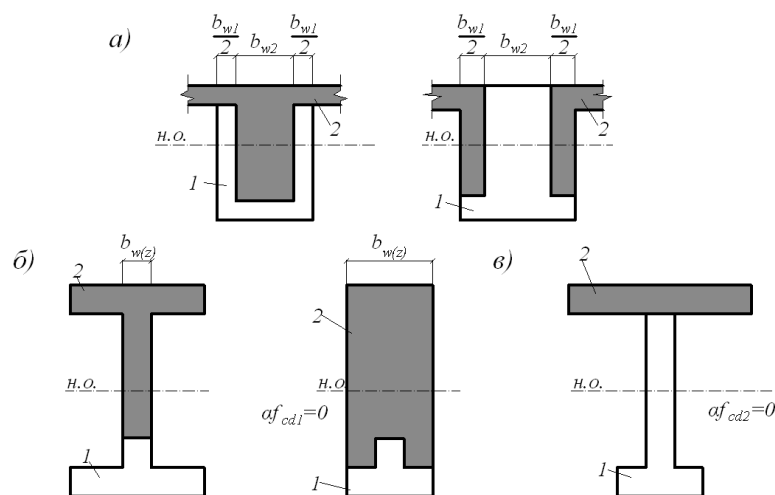
Рисунок 9.13 – Сборно-монолитные сечения
