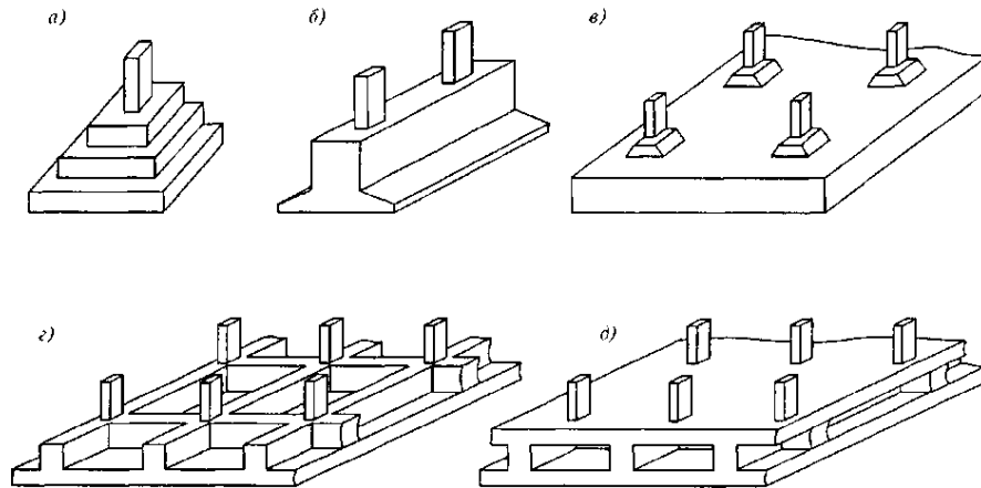
a - отдельный; б - ленточный; в, г, д - плитные: сплошной, ребристый и коробчатый
