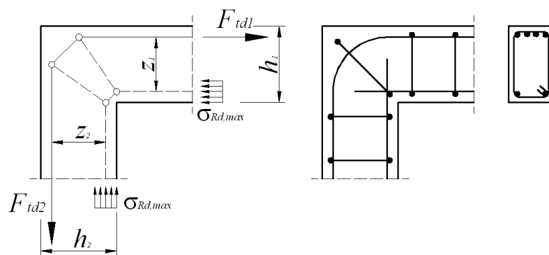
а) Почти равная высота колонны и балки
