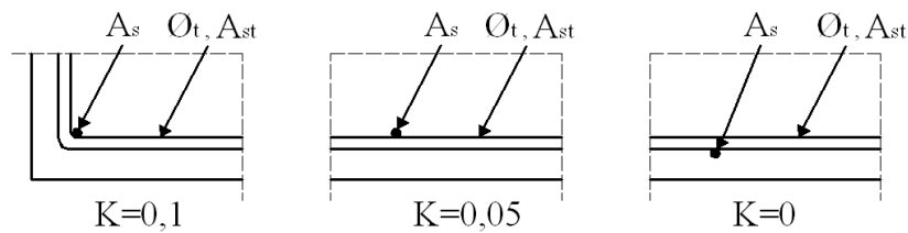
Рисунок 7.4 – Значения K для балок и плит
