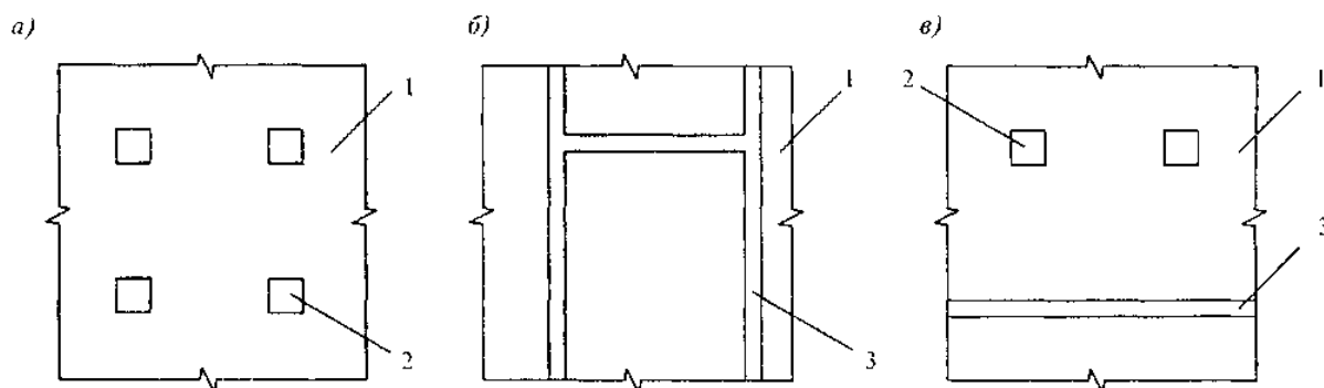
а - колонная КС; б - стеновая КС; в - смешанная КС; 1 - плита перекрытия; 2 - колонны; 3 - стены
