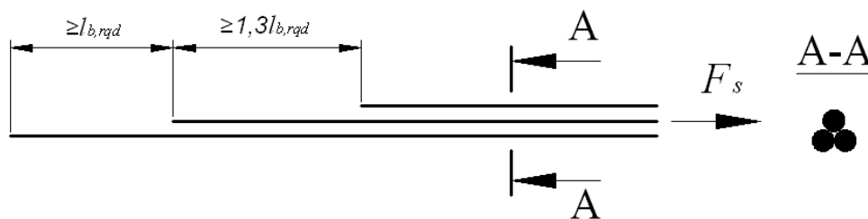
Рисунок 7.12 – Анкеровка стержней пучка, обрываемых ступенчато
