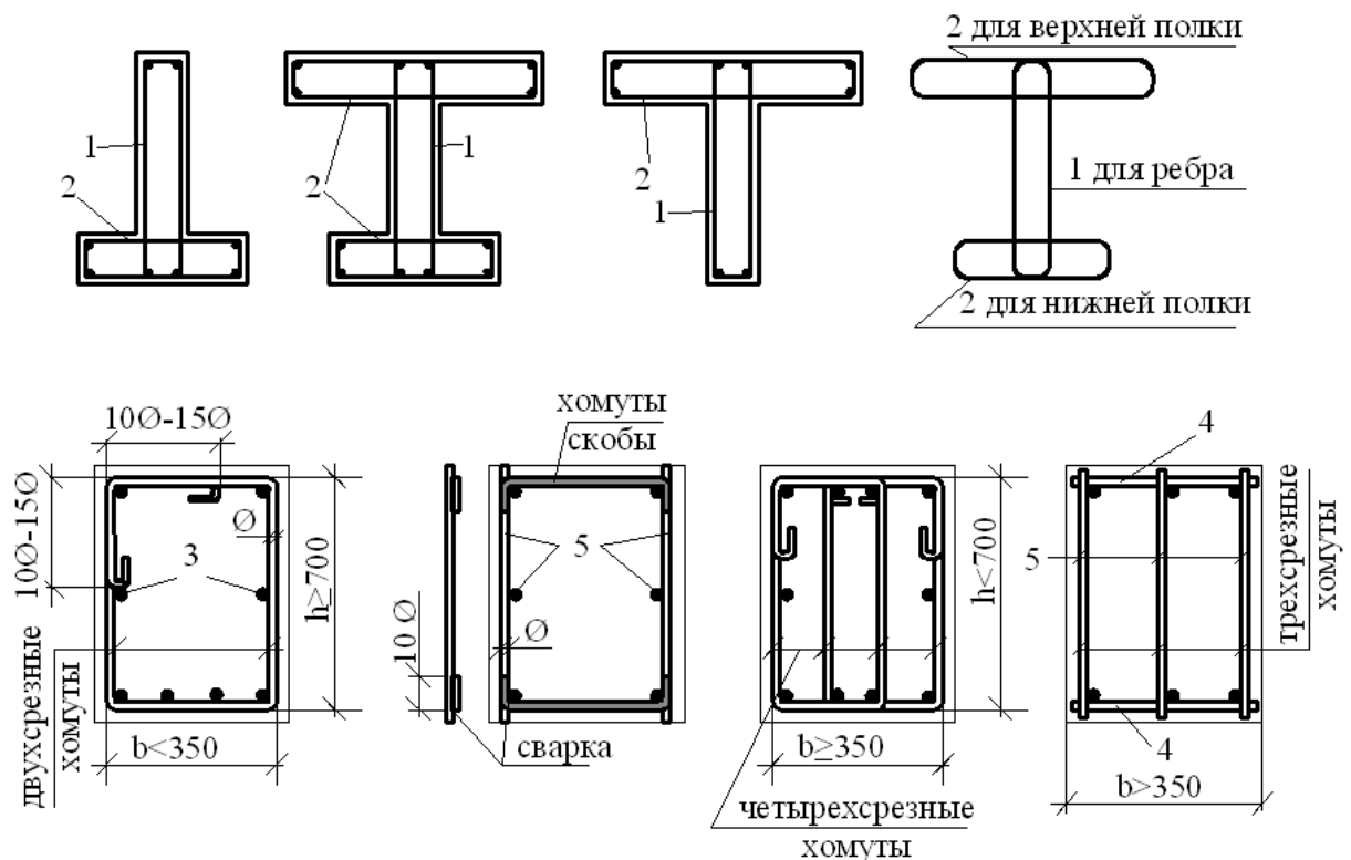
Рисунок 7.21 – Армирование элементов, работающих на изгиб с кручением
