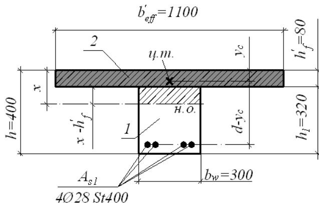
Плечо внутренней пары сил z = d - y_c
