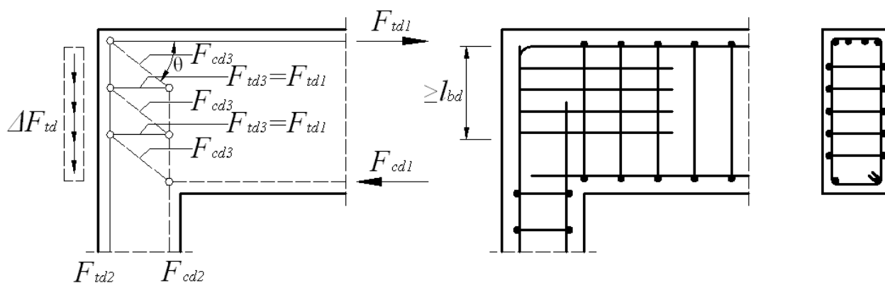
б) Значительно различающиеся высоты колонны и балки
