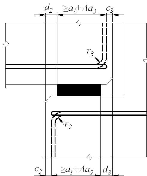
Рисунок 8.5 – Пример конструирования арматуры на опоре
