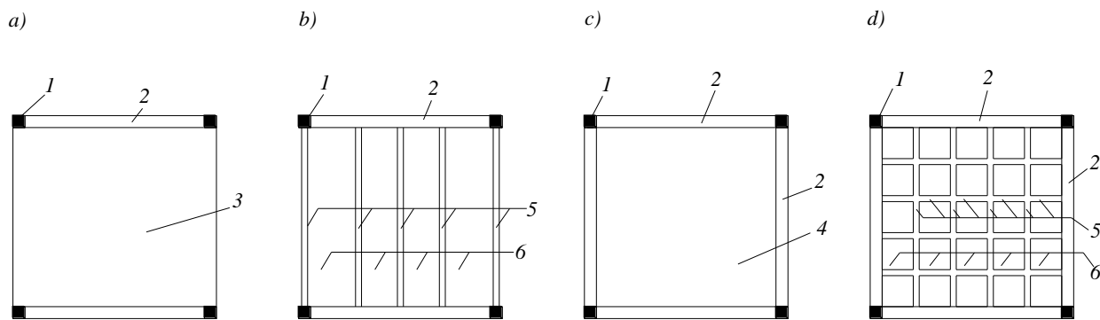
a, b - балки и стены в одном направлении; c, d - балки и стены в двух направлениях; 1 - колонны; 2 - балки или стены; 3 - плита сплошная или пустотная; 4 - плита сплошная, пустотная или кессонная; 5 и 6 - ребра и полки ребристой и кессонной плит
