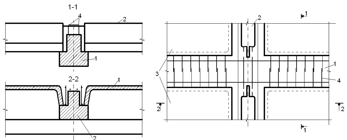
Рисунок 9.30 – Сопряжение балок и плит
