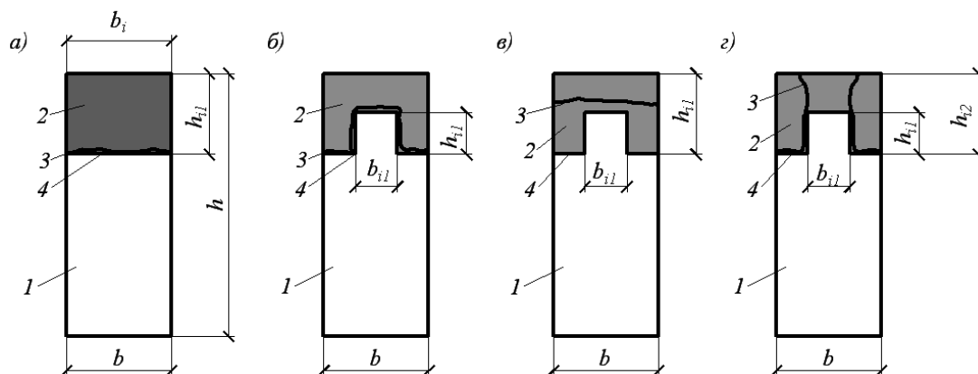
Рисунок 9.20 – Схемы расположения поверхностей сдвига, принимаемые для расчета контактного шва
