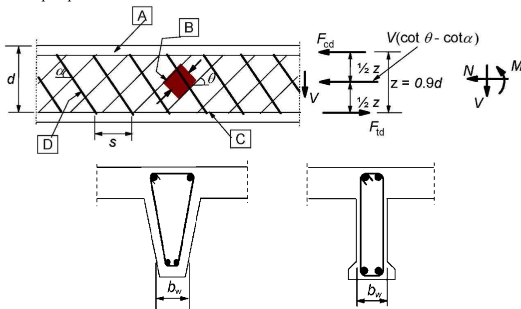
Рисунок 9.11 – К расчету прочности железобетонных элементов при действии поперечной силы на основе стержневой модели
