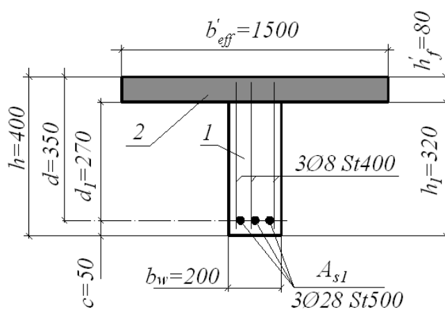
Рисунок Г.10 – К расчету прочности сечения составной балки по наклонной трещине
