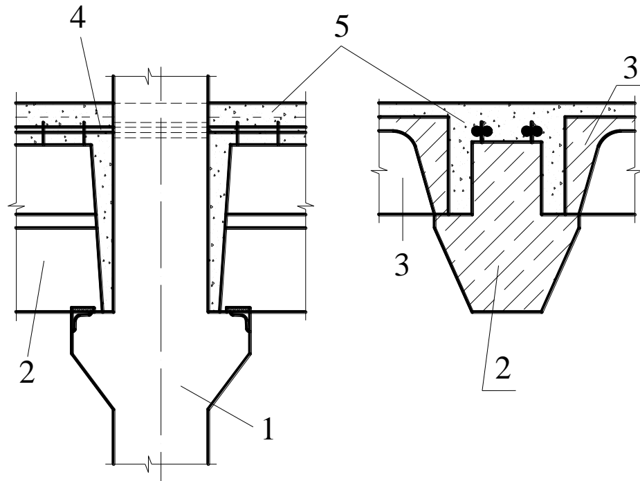
1 – колонна; 2 – сборные ригели; 3 – сборные плиты; 4 – надпорная арматура ригелей; 5 – монолитный бетон
