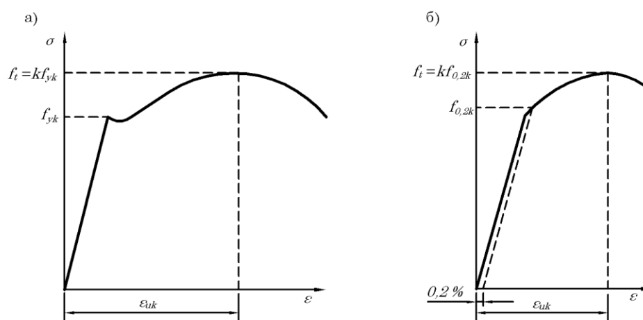
а – для горячекатаной стали; б – для холодноотянутой стали
