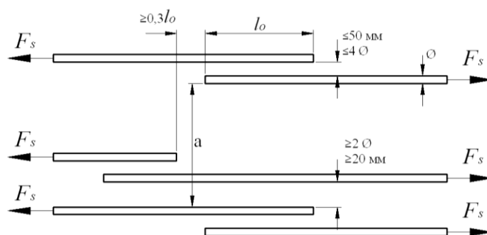
Рисунок 7.7 – Соседние соединения в нахлестку
