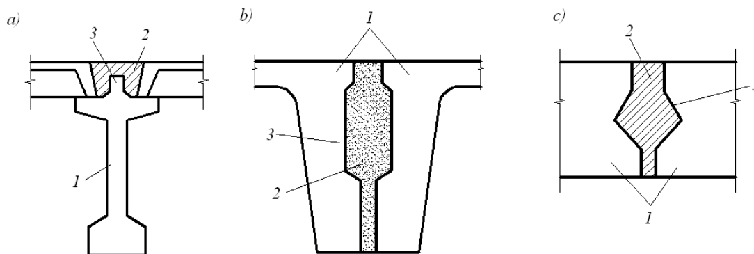
1 – сборный элемент; 2 – монолитный бетон; 3 – продольный выступ или паз
