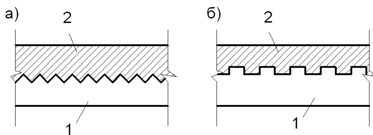
1 – сборный элемент; 2 – монолитный бетон
