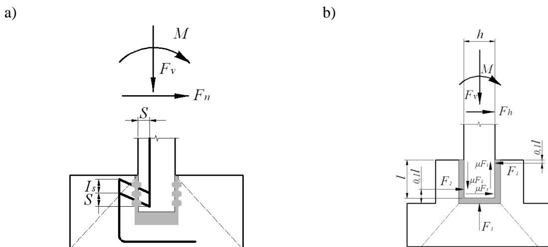
Рисунок 8.7 – Фундаменты стаканного типа: а – со шпоночной поверхностью; б – с гладкой поверхностью
