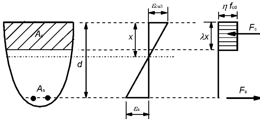
Рисунок 9.2– Равномерное распределение напряжений по высоте эффективной сжатой зоны сечения
